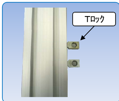
1. Tロックを溝に入れる。
