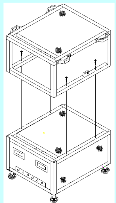
分割図
